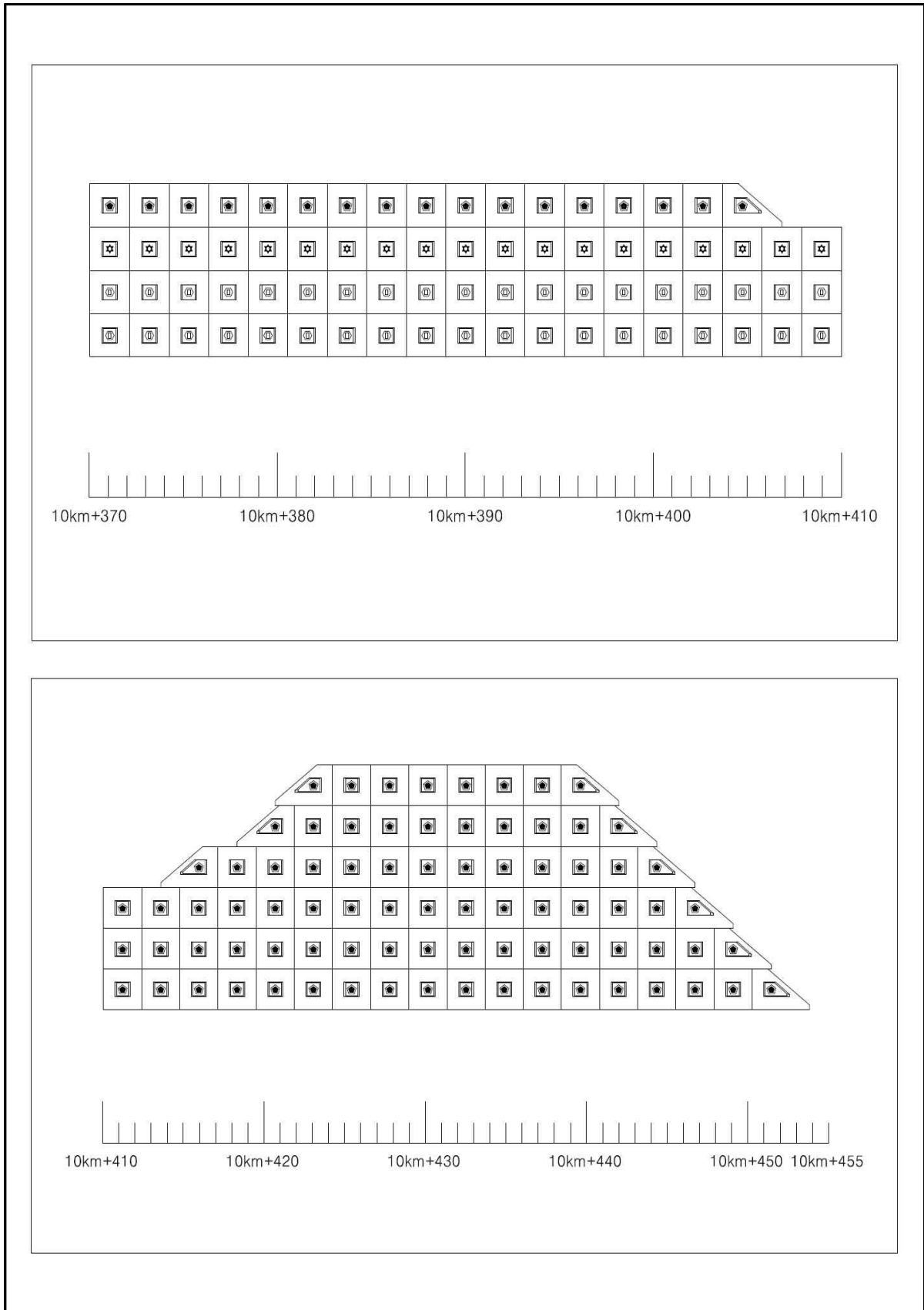
【그림 10.1.4】 전개도(계속) 【그림 10.1.4】 전개도(계속)
