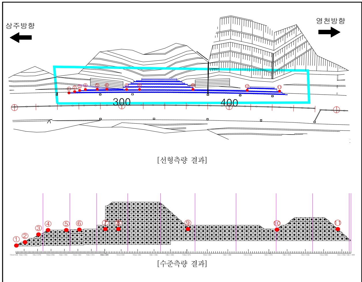
【그림 10.3.4】 선형 및 수준측량 결과
